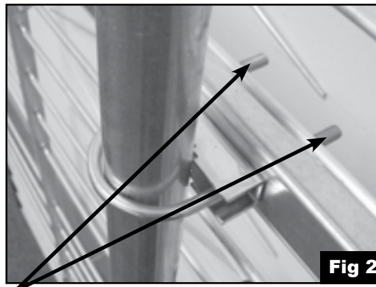
U-bolt must be secured with bolts thru antenna. Tornillos en forma de U deben ser asegurados con cerrojos a través de la antena.
